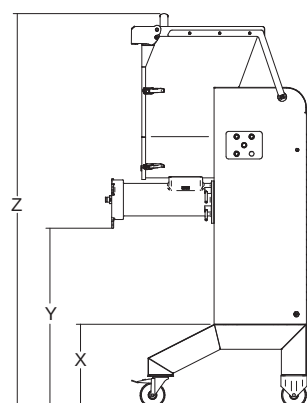
MASTER 90 Y12 gambe alte opzionali optional high legs X: 333 mm Y: 717 mm Z: 1575 mm
